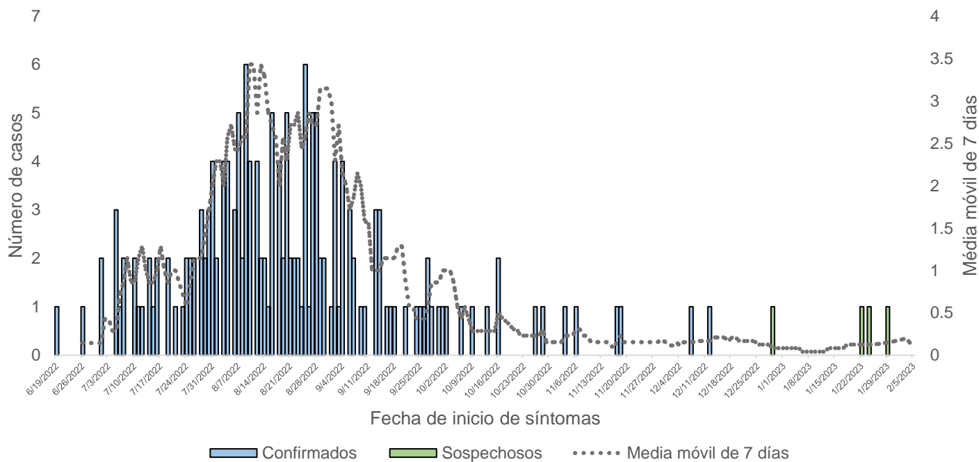
Gráfica 1. Curva epidémica de casos confirmados y sospechosos para virus Orthopox detectados en Puerto Rico, por fecha de inicio de síntomas (N=177).
