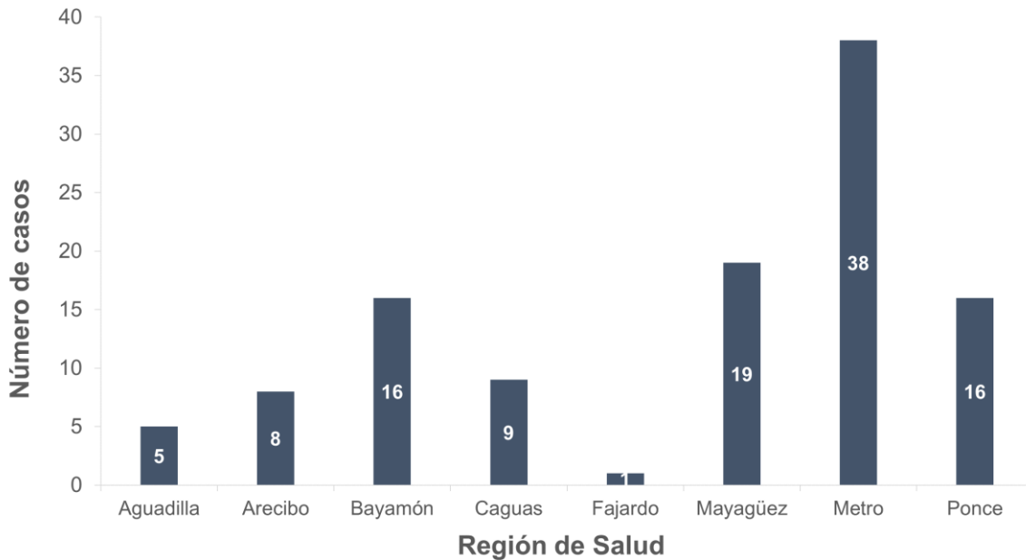
Gráfica 3. Distribución de incidencia acumulada de Enfermedades Transmisibles por Alimentos y/o Agua por región de salud, semana epidemiológica 18, 2023 (N=112)
