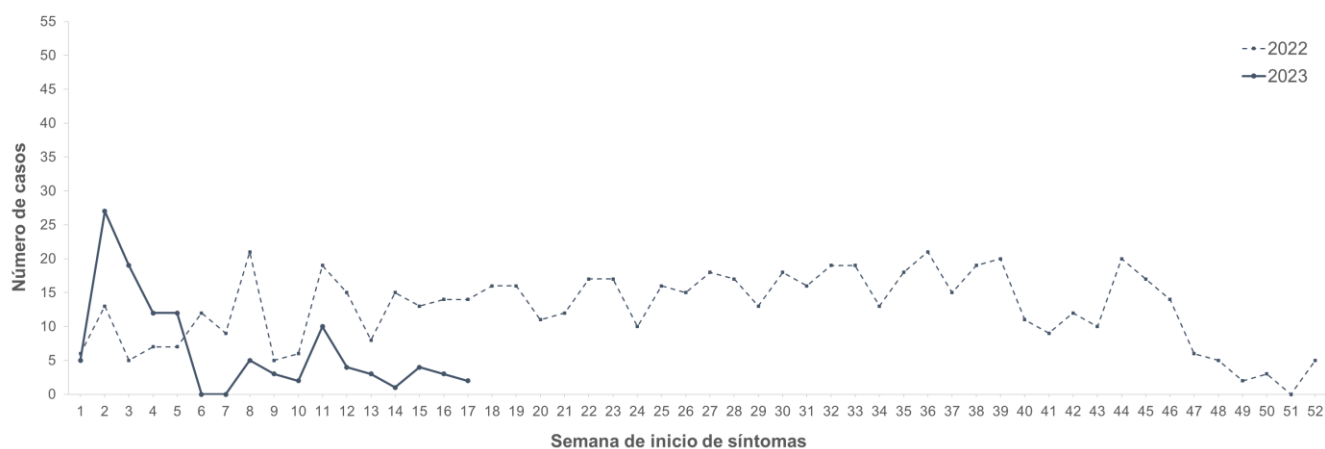
Gráfica 1. Incidencia acumulada de Enfermedades Transmisibles por Alimentos y/o Agua por semana epidemiológica, semana epidemiológica 18, 2023 (N=112)
