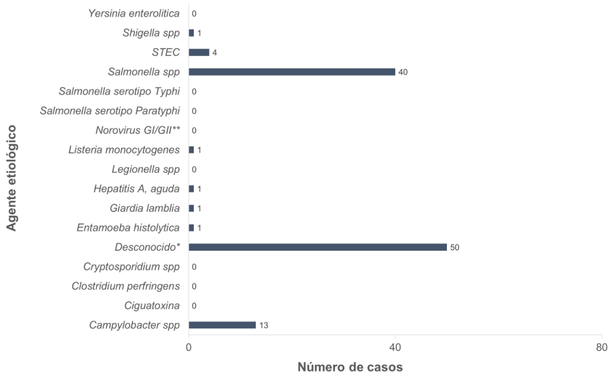
Gráfica 4. Incidencia acumulada de Enfermedades Transmisibles por Alimentos y/o Agua según el agente etiológico, semana epidemiológica 18, 2023 (N=112)
