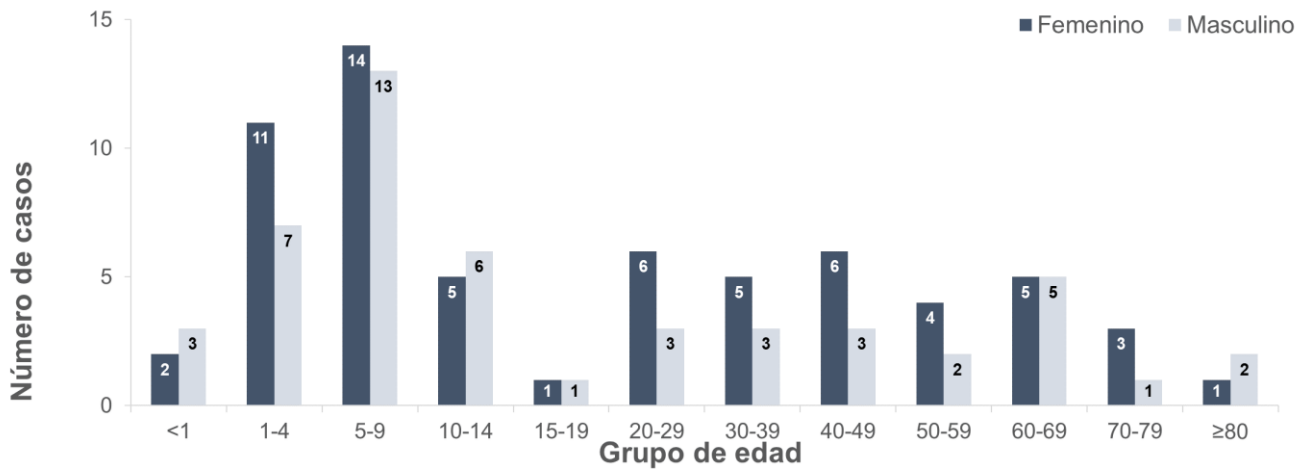
Gráfica 2. Incidencia acumulada de Enfermedades Transmisibles por Alimentos y/o Agua por sexo y grupo de edad, semana epidemiológica 18, 2023 (N=112)
