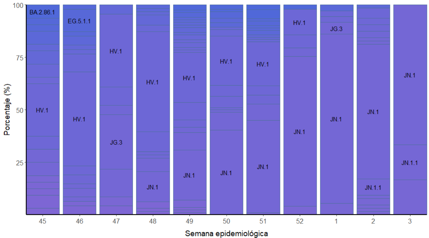
Gráfica 7. Proporción de linajes y sublinajes de variantes de SARS-CoV-2 de preocupación, interés o bajo monitoreo de Puerto Rico reportadas al Sistema de Vigilancia Genómica, por semana epidemiológica.
