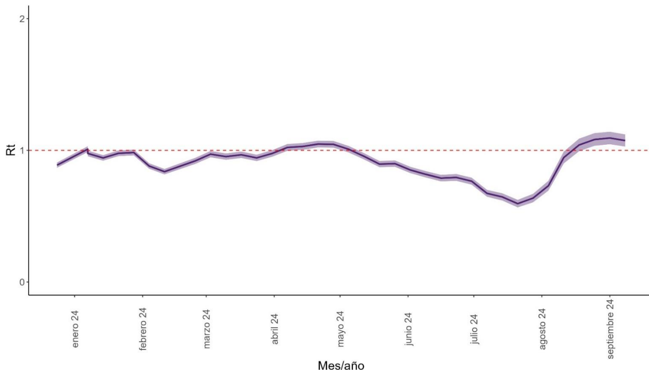
Gráfica 10. Estimados de R_t para casos de Influenza en Puerto Rico, 31 de diciembre de 2023 al 28 de septiembre de 2024. Parámetro: media = 2.5 días y desviación estándar = 2 días
